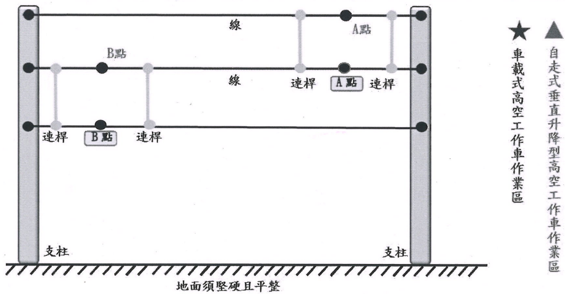
立面圖
